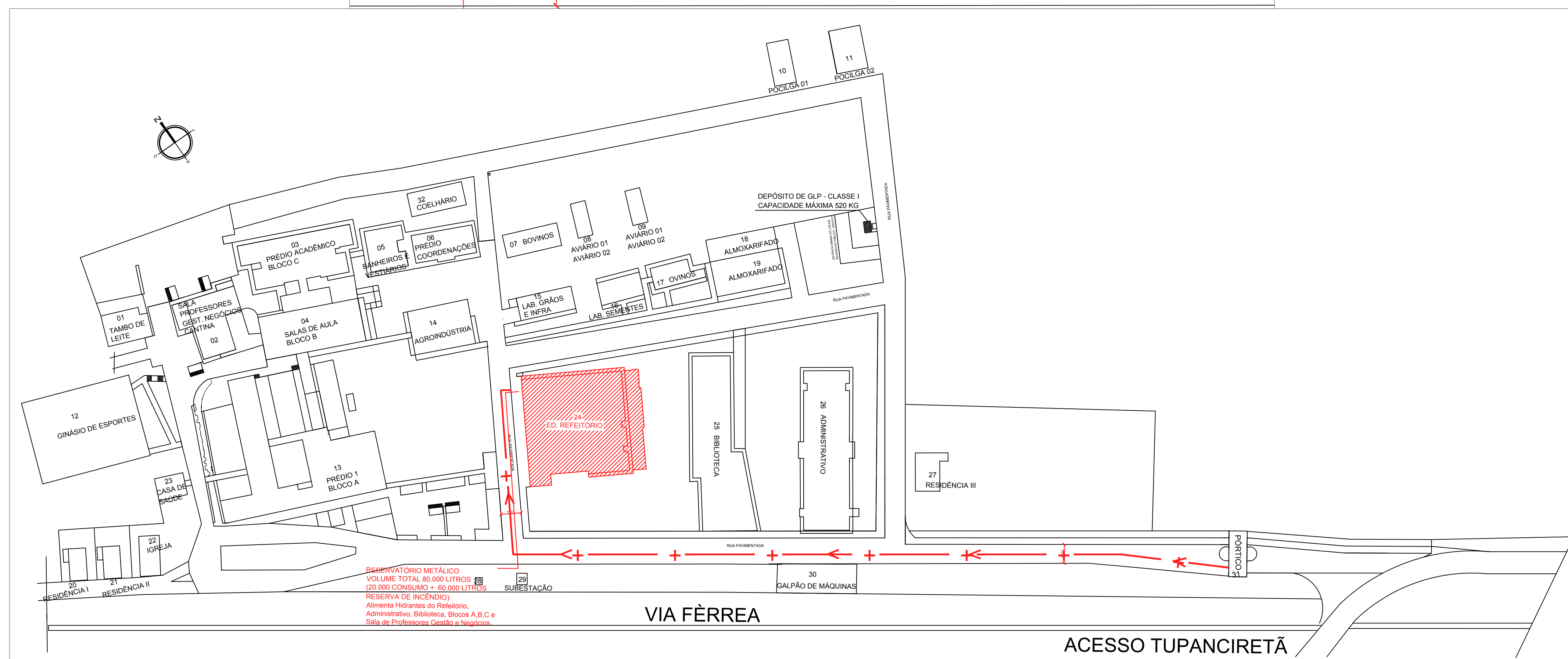
PLANTA DE LOCALIZAÇÃO ESCALA: 1/500
